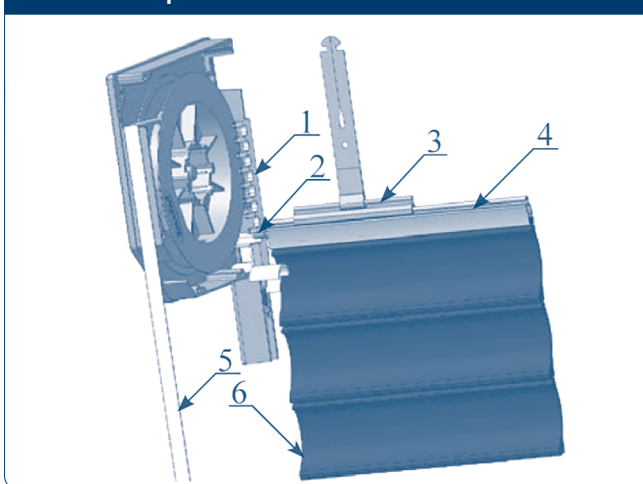
Рис. 8.2.1. Закрытое положение
