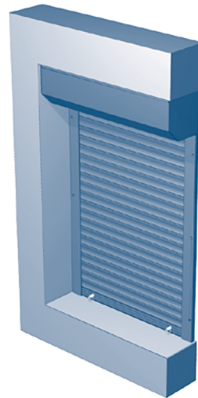
Рис. 6.2.2. Встроенный монтаж, короб наружу
